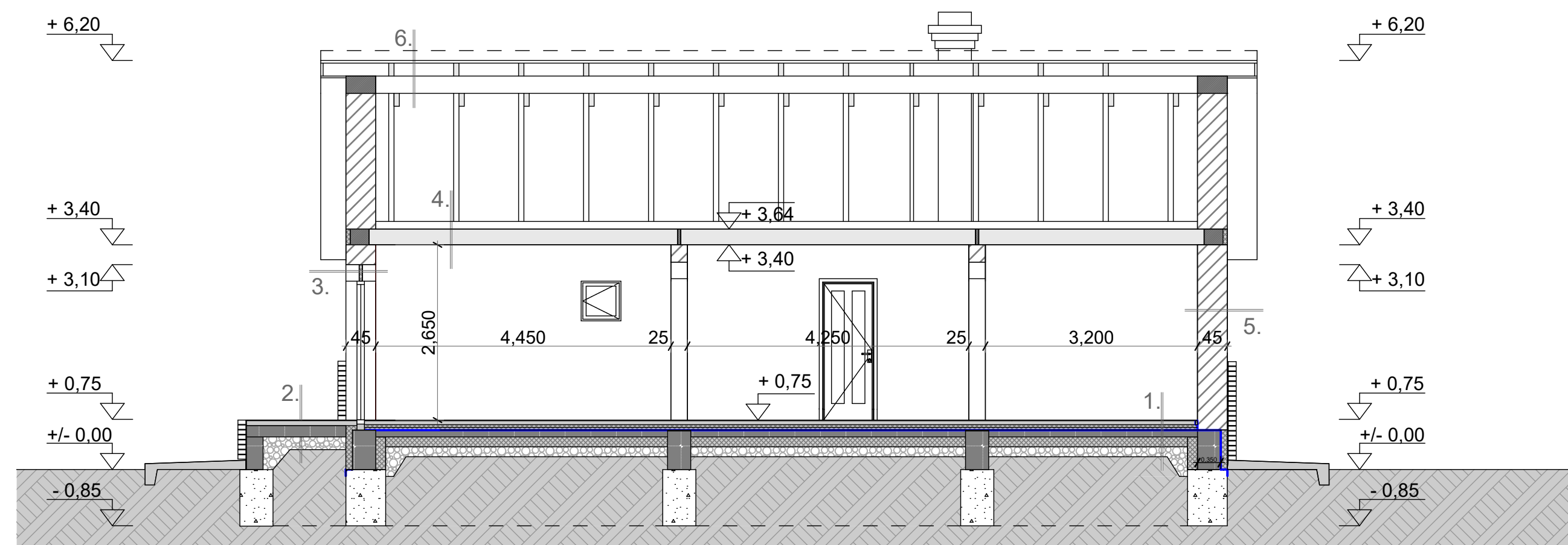
B - B metszet
