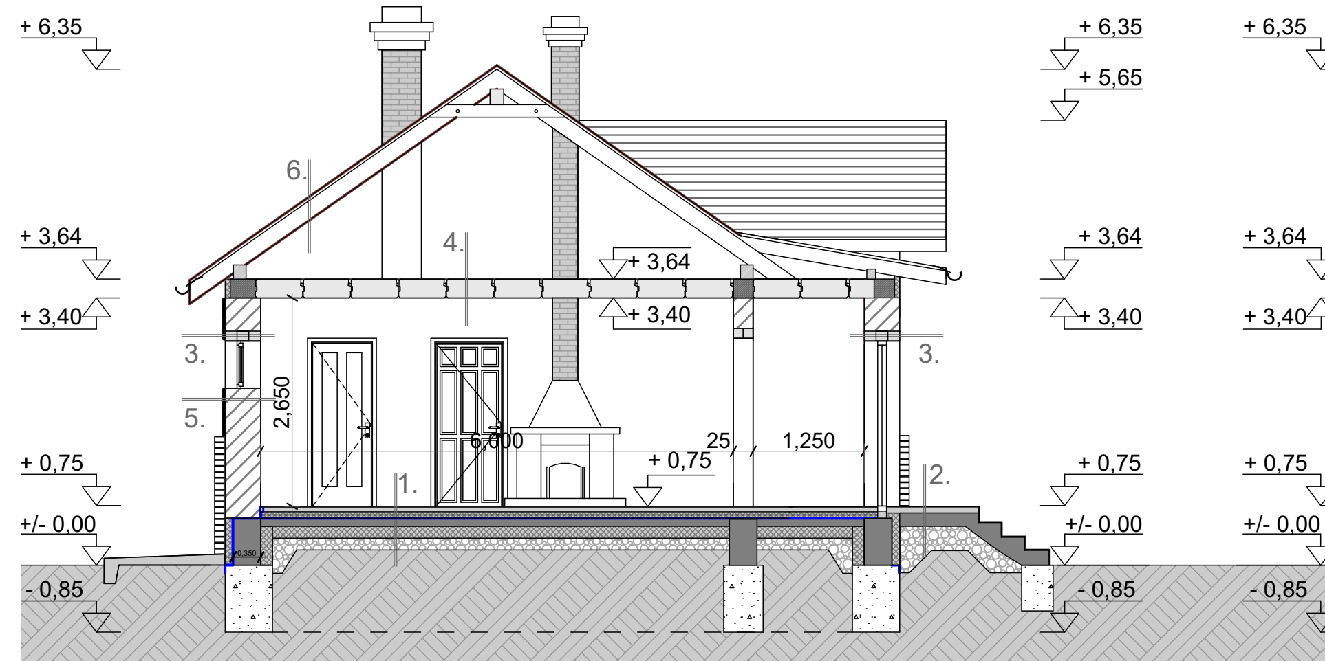
A - A metszet
